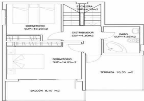
Planta Primera
