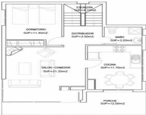
Planta Baja
