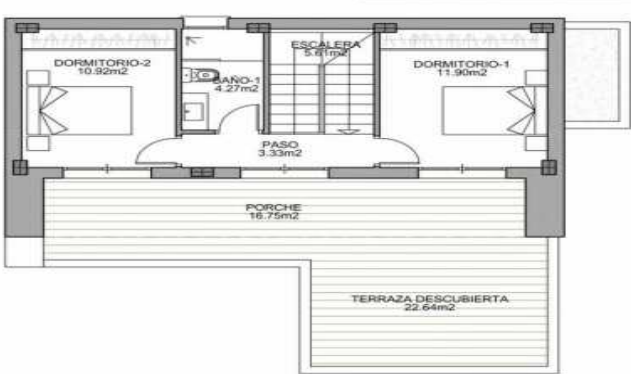
PLANTA PRIMERA
